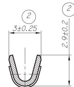
CORTE A-A
